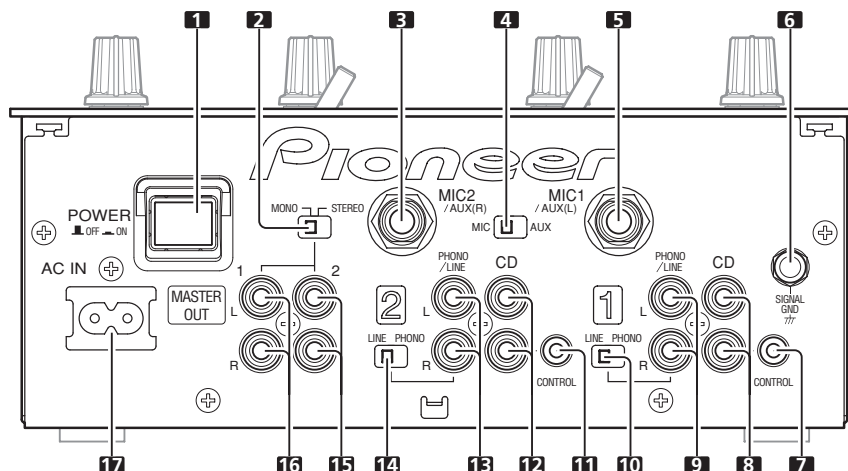
Pannello posteriore
